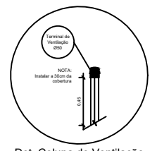
Det. Coluna de Ventilação Escala 1/10
