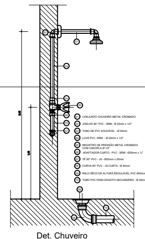
Det. Chuveiro Escala 1/25
