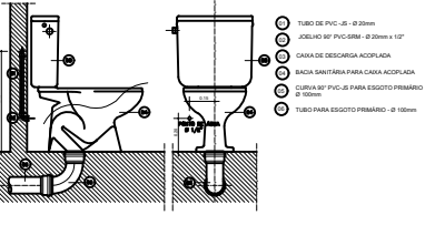
Det. Vaso sanitário c/ Cx acoplada Escala 1/25
