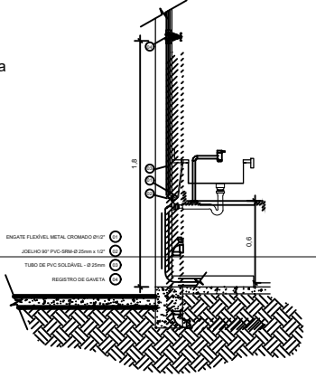
Det. Pia Escala 1/25
