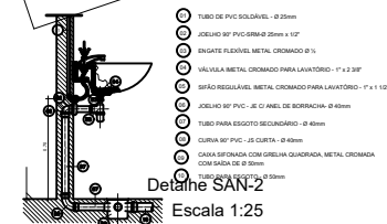
Det. Lavatório Escala 1:25
