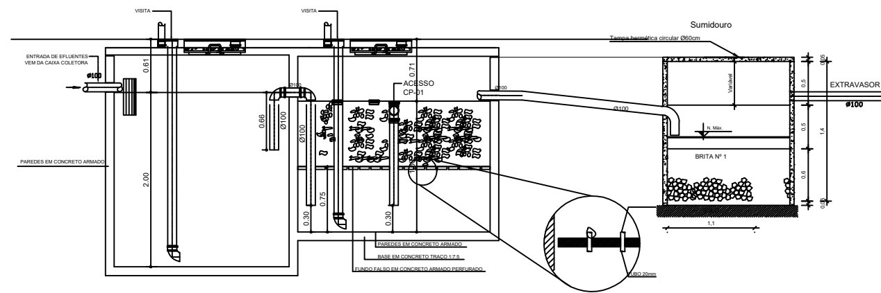
DETALHE FOSSA/FILTRO/SUMIDOURO escala.....1:25
