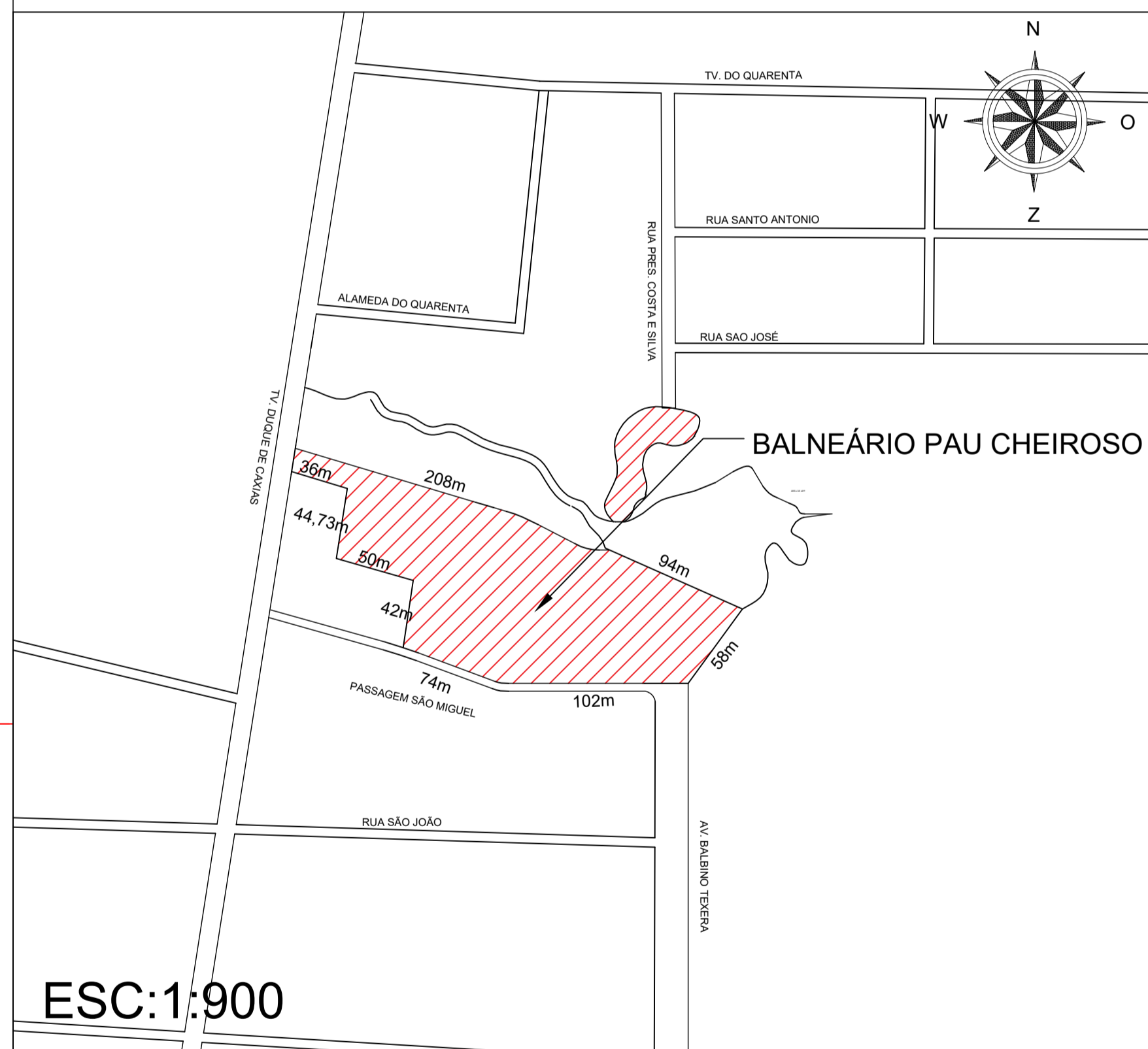
PLANTA DE SITUAÇÃO
