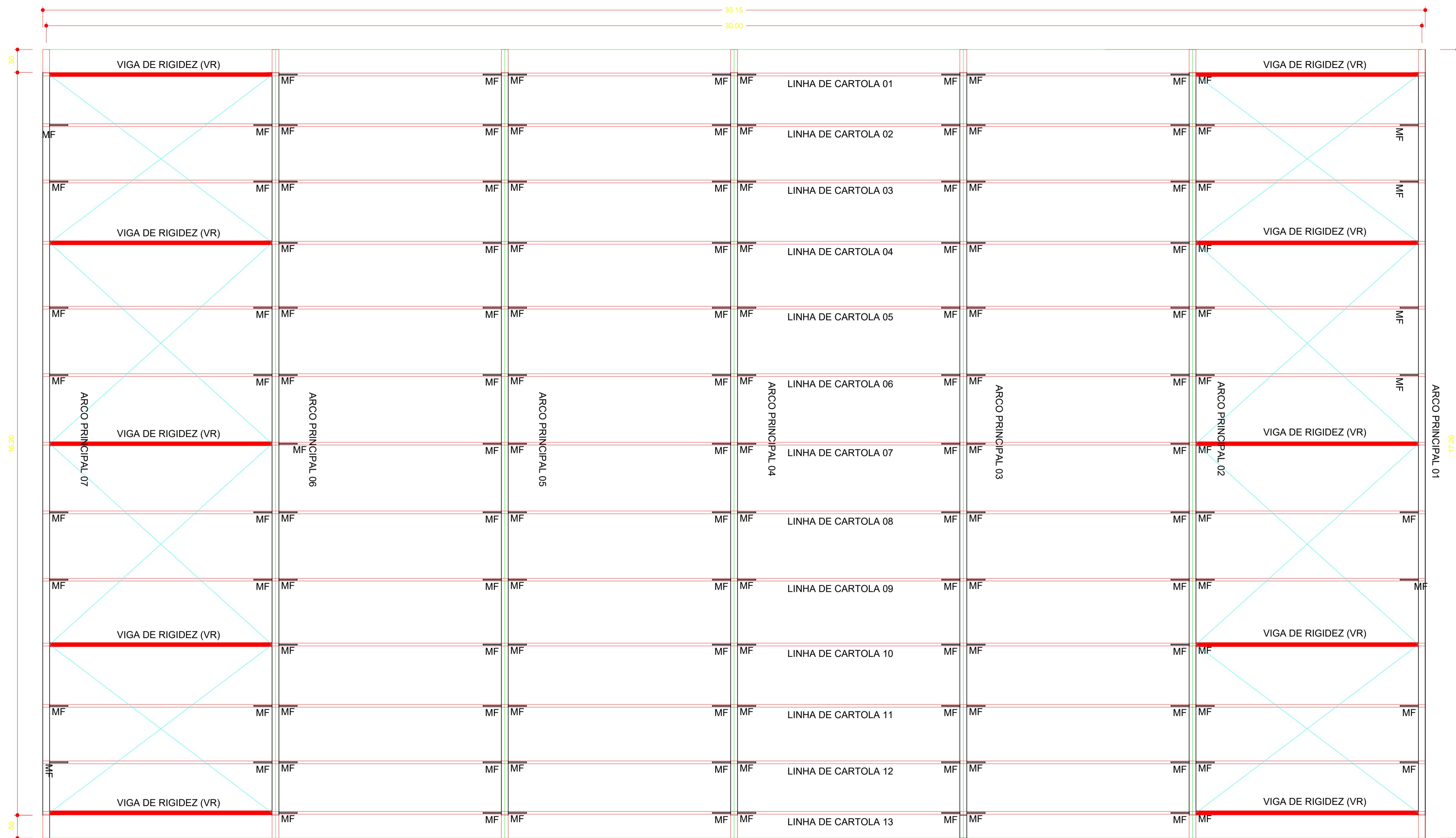
PLANTA DA COBERTURA ESCALA: 1/100
